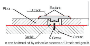
T-MOLDING
